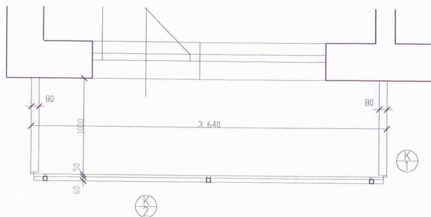
PŮDORYS BALKÓNU - Nový stav
