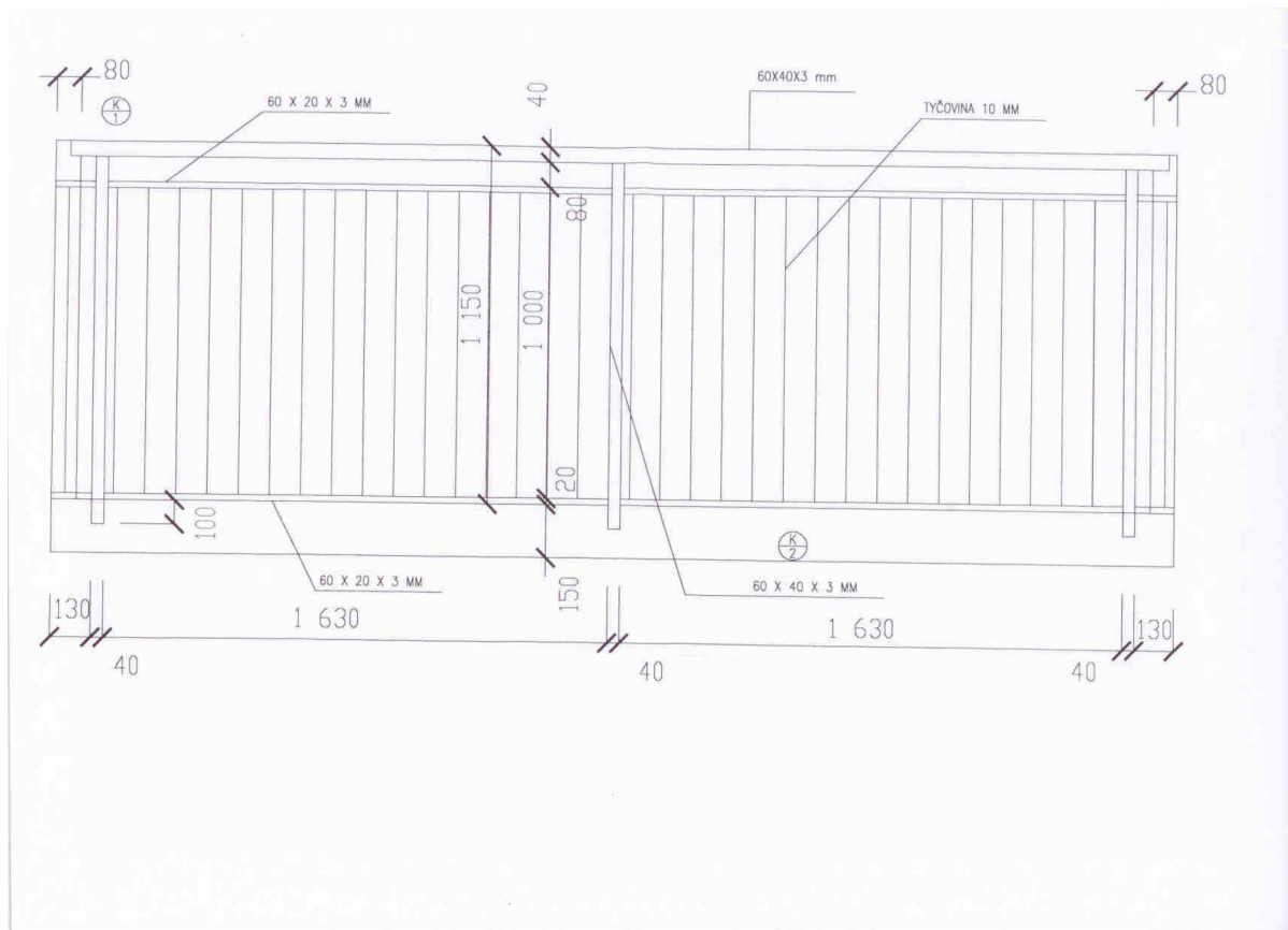
Čelní pohled balkónu – nový stav
