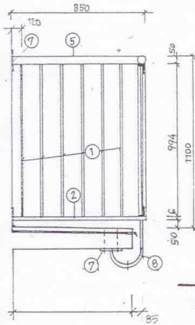
Pohled (P2) Měř. 1 : 20
