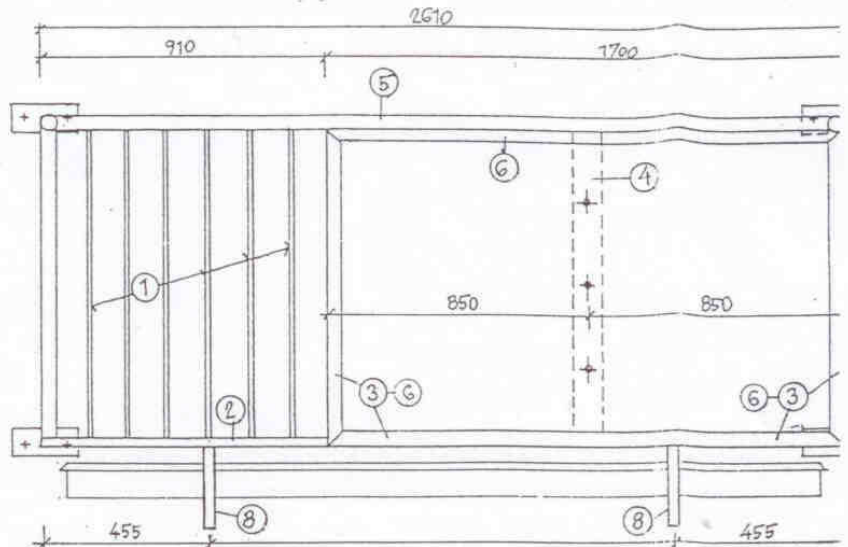
Pohled (P1) Měř. 1 : 20
