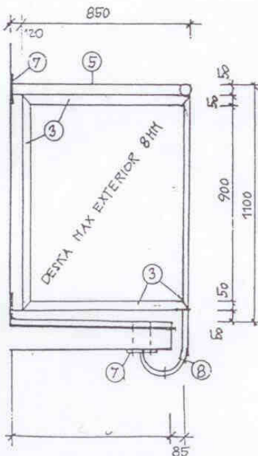
Pohled (P3) Měř. 1 : 20
